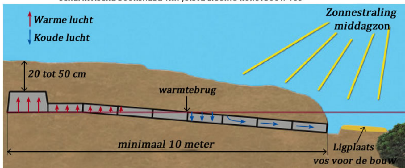
SCHEMATISCHE DOORSNEDE VAN JUISTE LIGGING KUNSTBOUW VOS
